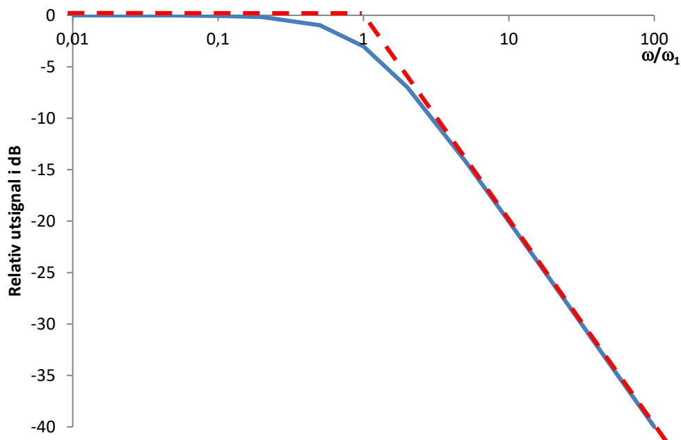
Fig. 4. Överföringskaraktistik för ett första ordningens lågpassfilter. Uppmätta värden (blå kurva) och asymptotisk approximation (streckad, röd kurva).
